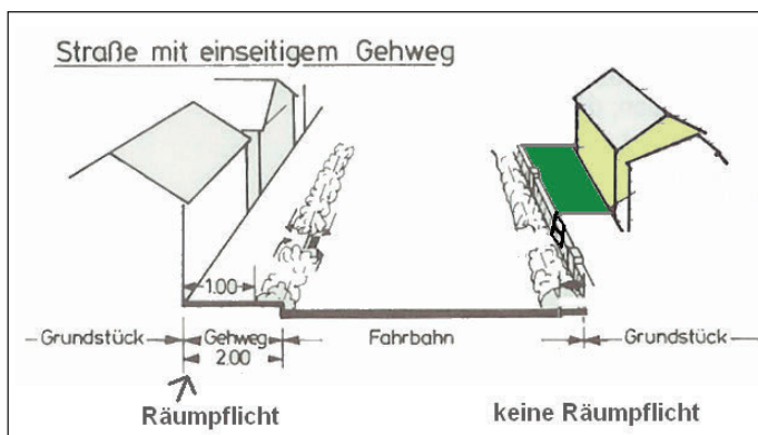
Abb. 1 Straße mit einseitigem Gehweg - Räumpflicht einseitig!
